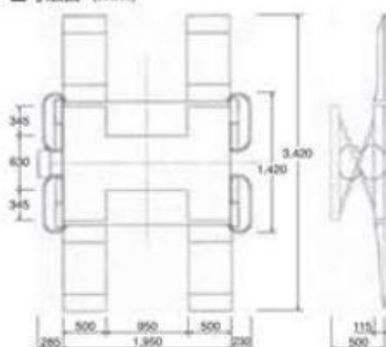
■寸法図 (mm)
